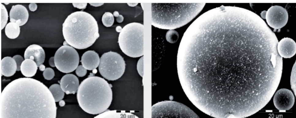
Внешний вид полых стеклянных микросфер. Снимок с микроскопа при 50-ти-кратном увеличении
