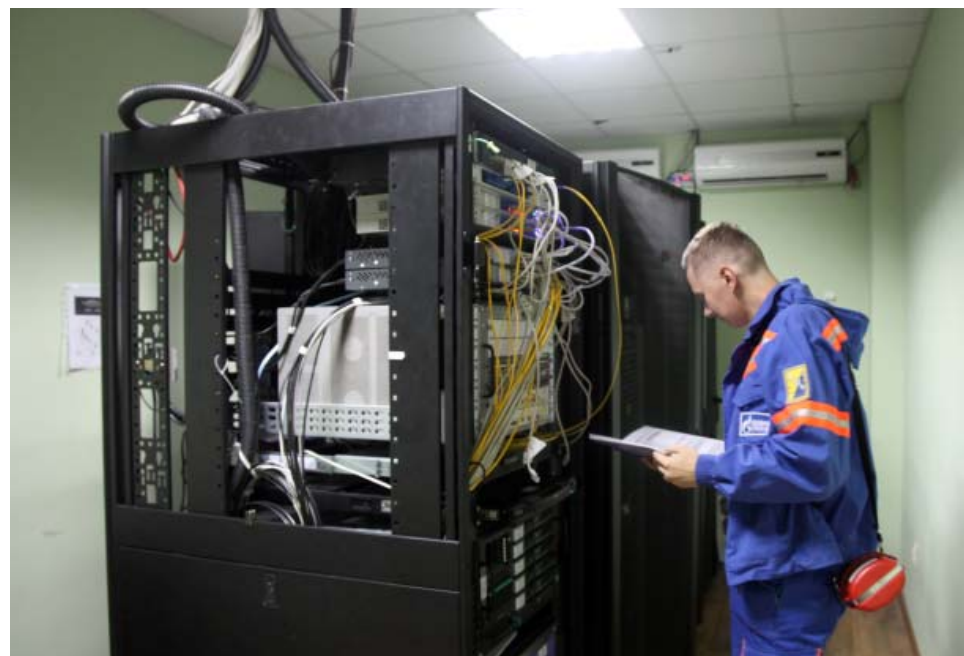
Электромонтёр линейных сооружений Алексей Горюков осуществляет визуальный осмотр и техническое обслуживание оборудования серверной
